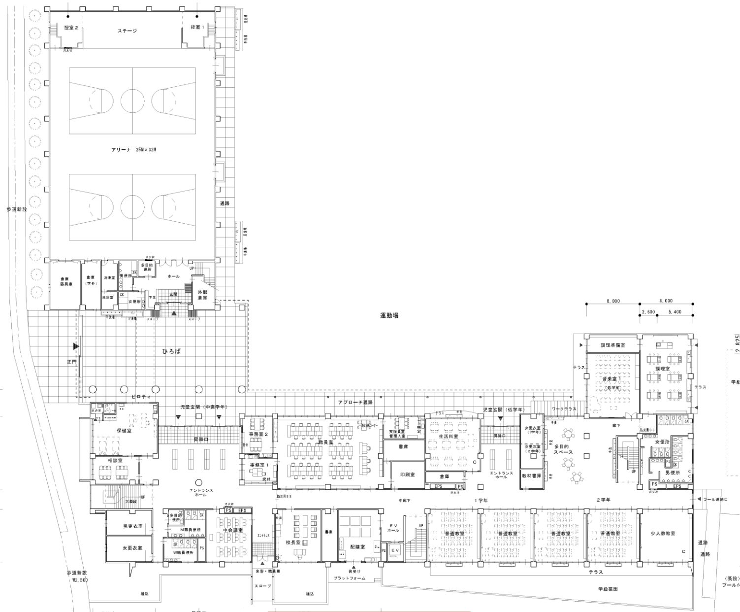
1F 平面図
