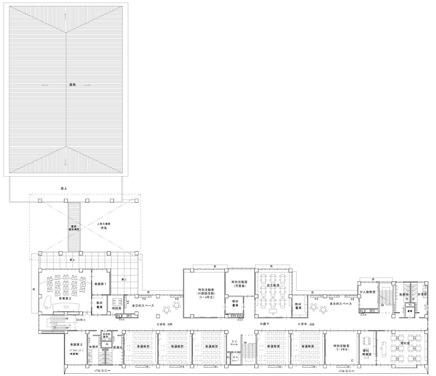
3F 平面図
