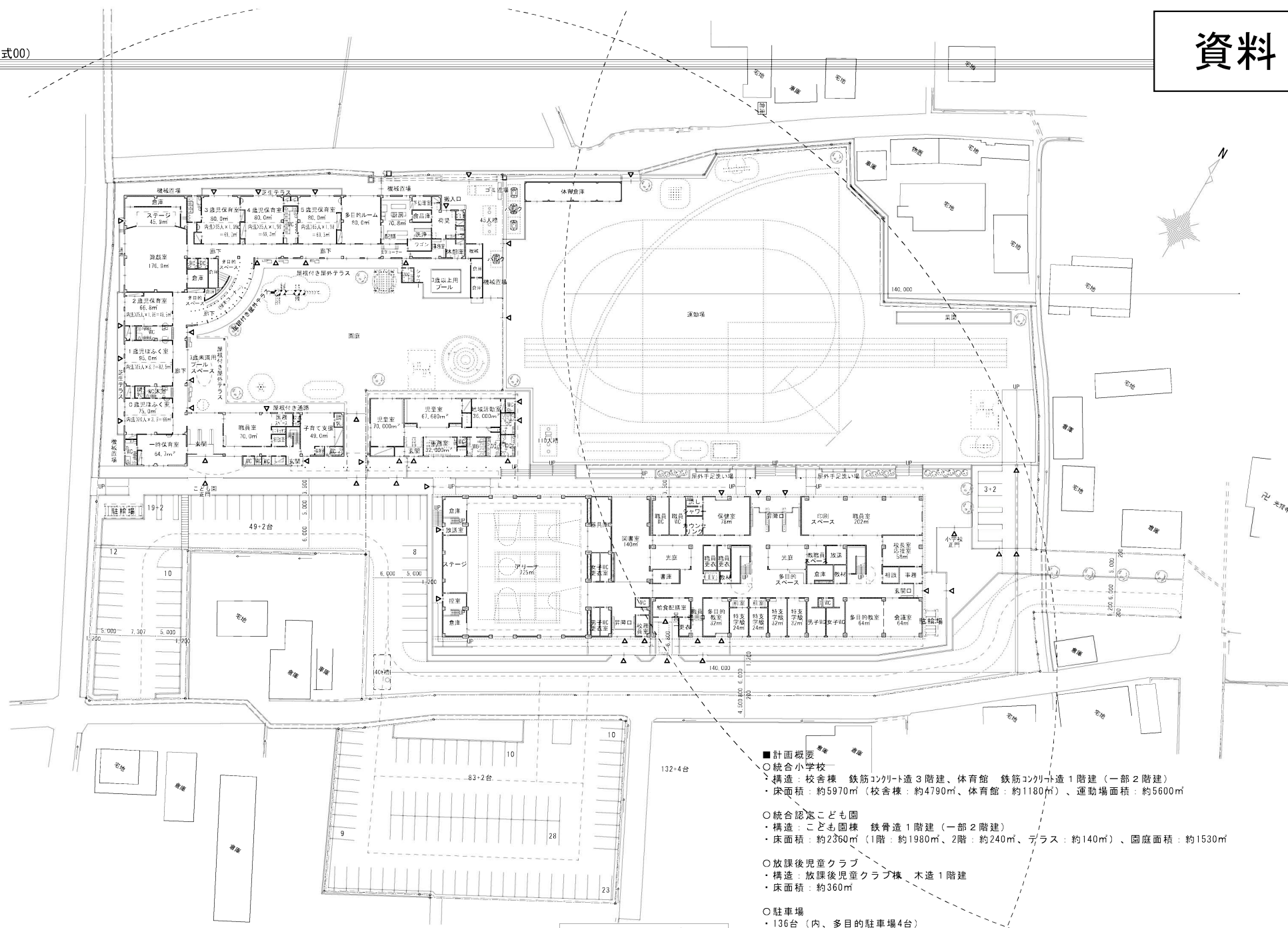
配置図 A3:1/700
